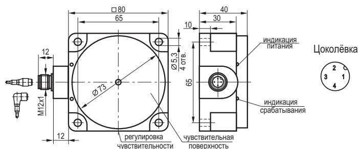
Габаритный чертеж
